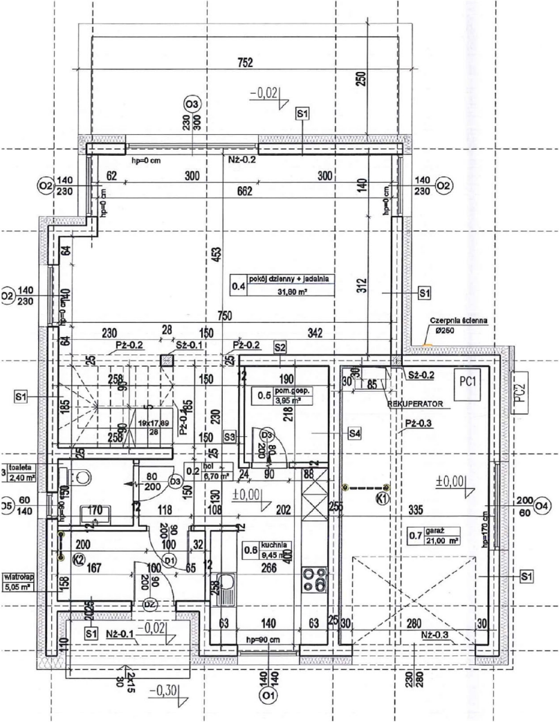
RZUT PARTERU
