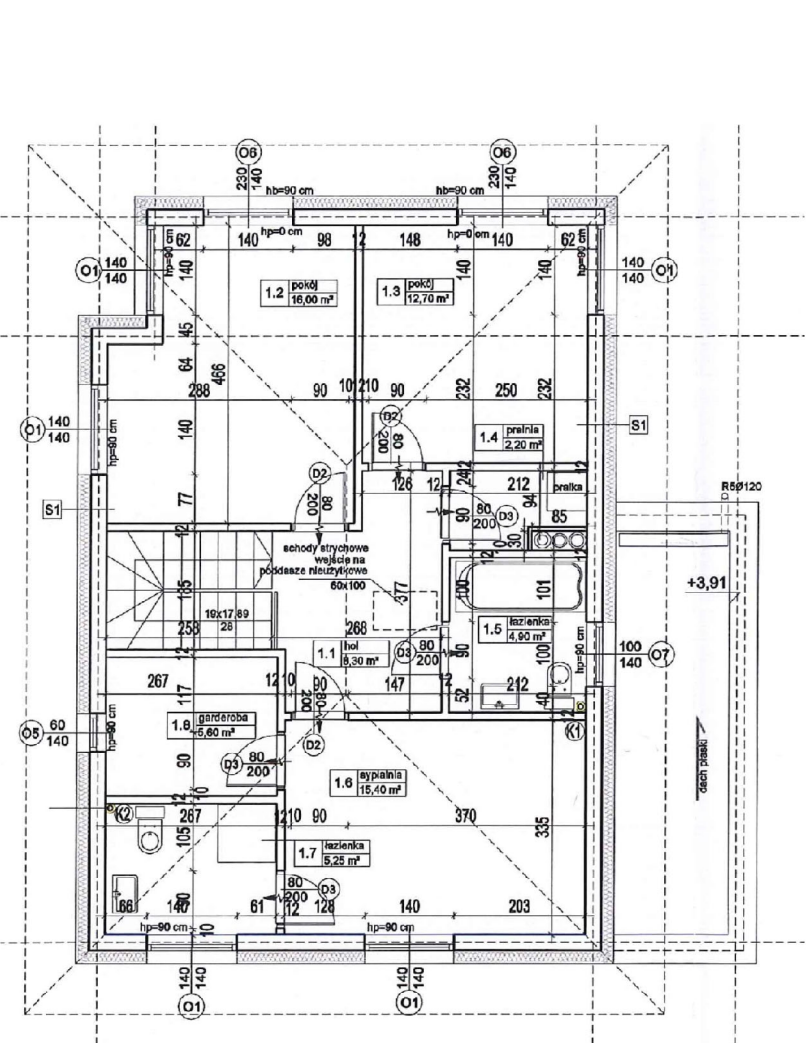
RZUT PIĘTRA
